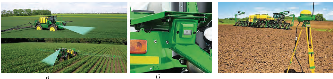
Рисунок 10 – Ілюстрація системи корекції положення агрегата «Guidance Radio RTK» фірми «Deere & Company» [Radio RTK 900, 2023]
