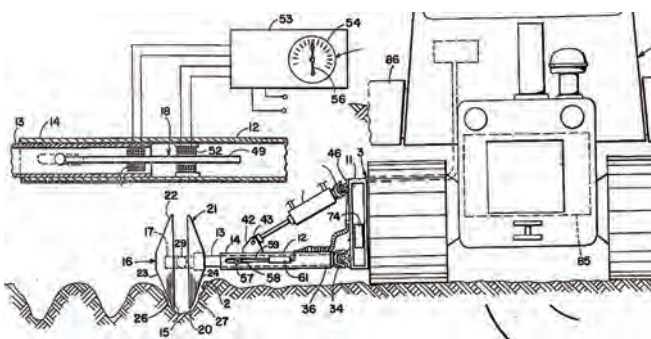
Рисунок 4 – Схема «Системи ведення гусеничних тракторів» з використанням борозни на поверхні ґрунту за патентом US4298084A - Guidance system for tracklaying tractors 1980 [Newell, 1980]
