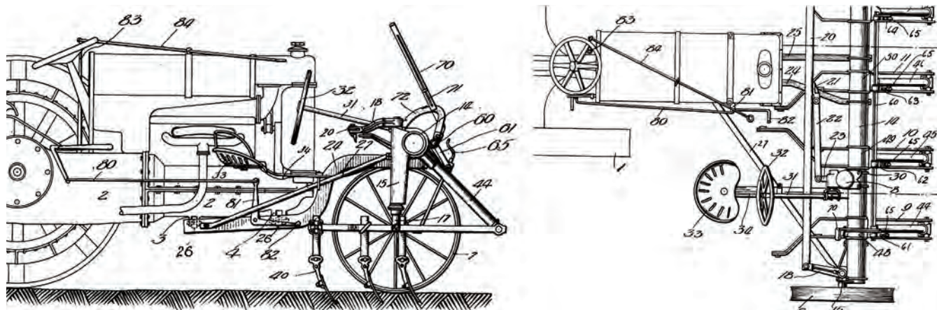
Рисунок 2 – Засіб коригування положення знаряддя на поверхні поля за патентом «Навісне обладнання для тракторів» [Rose, 1922]
