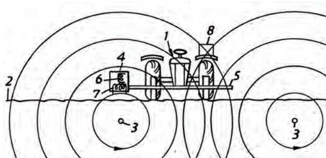
Рисунок 3 – Схема використання електромагнітного випромінювання від дроту у товщі ґрунту за патентом «Системи ведення колісного засобу» US3679019A - Vehicle guidance systems (1970) [Hobday, Hobday, 1970]
