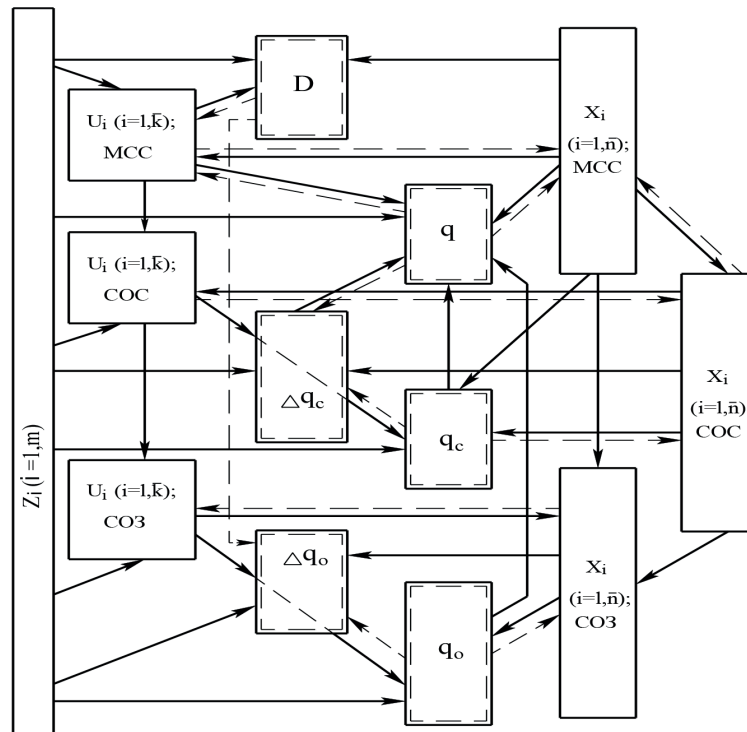
Рисунок 1 – Графічна модель молотарки барабанного типу на рівні показників призначення:
