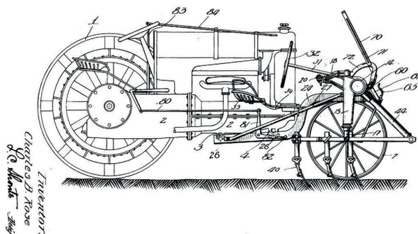
Рисунок 5 – Технічне рішення за патентом «Навісне обладнання для тракторів» US1472888 [14]
