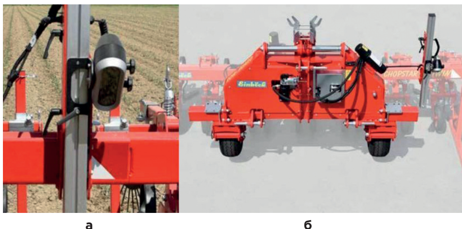
Рисунок 13 – Основні елементи Camera steering system ROW-GUARD фірми Einbock GmbH&Co [31]: а – відеокамера з двома об'єктивами високої чіткості з різною експозицією для поліпшення роботи зі зміною умов світла; б – система зміщення культиватора відносно рядка рослин
