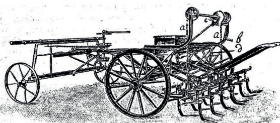
Рис. 84. Полольник завода в Эрцгебирге.
