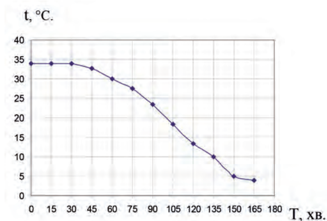
Рисунок 5 – Графік залежності температури молока (t) від тривалості охолодження (T)
